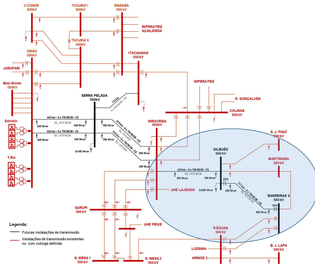
Figura 4-9 - Reforços na interligação Norte-Nordeste – Solução mitigadora dos atrasos de obras
