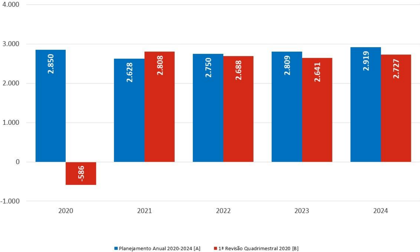
SIN. Variações anuais da carga de energia (MWmédio)
