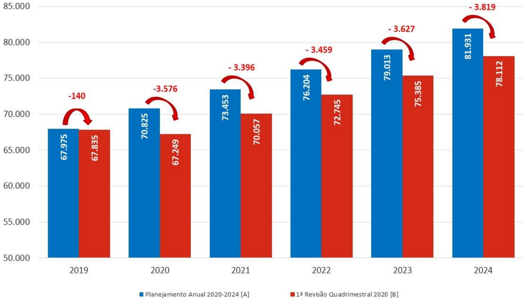
SIN. Carga de energia (MWmédio)
