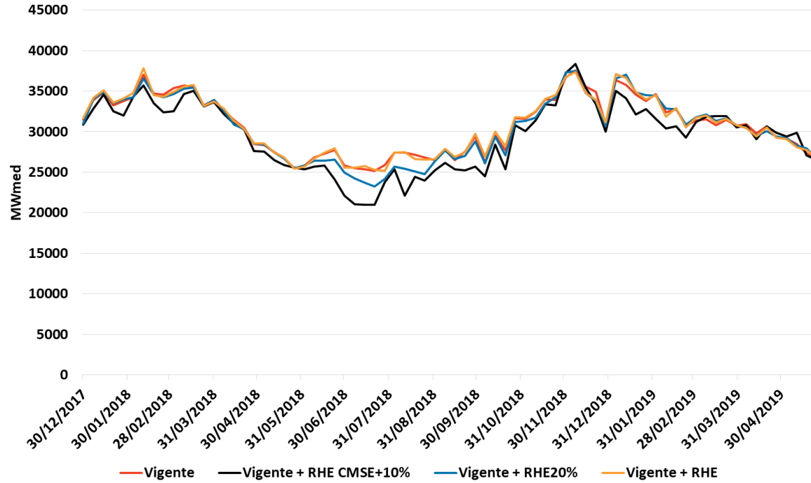
GH Sudeste
