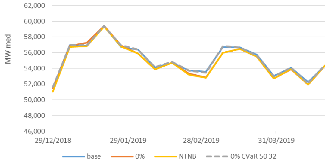
GH SIN
