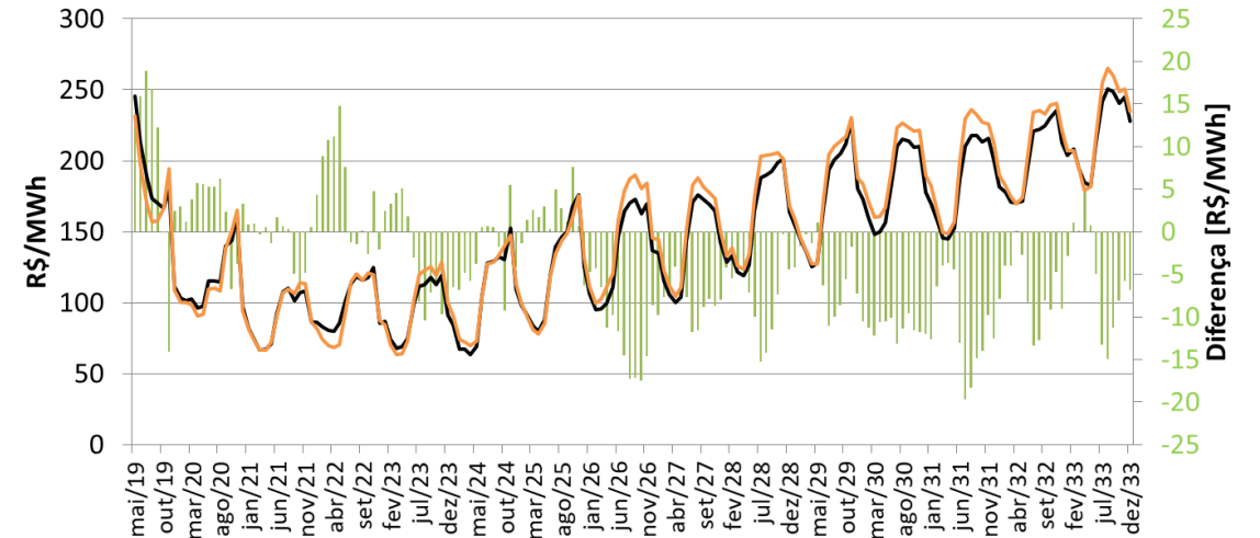
CMO - NORTE
