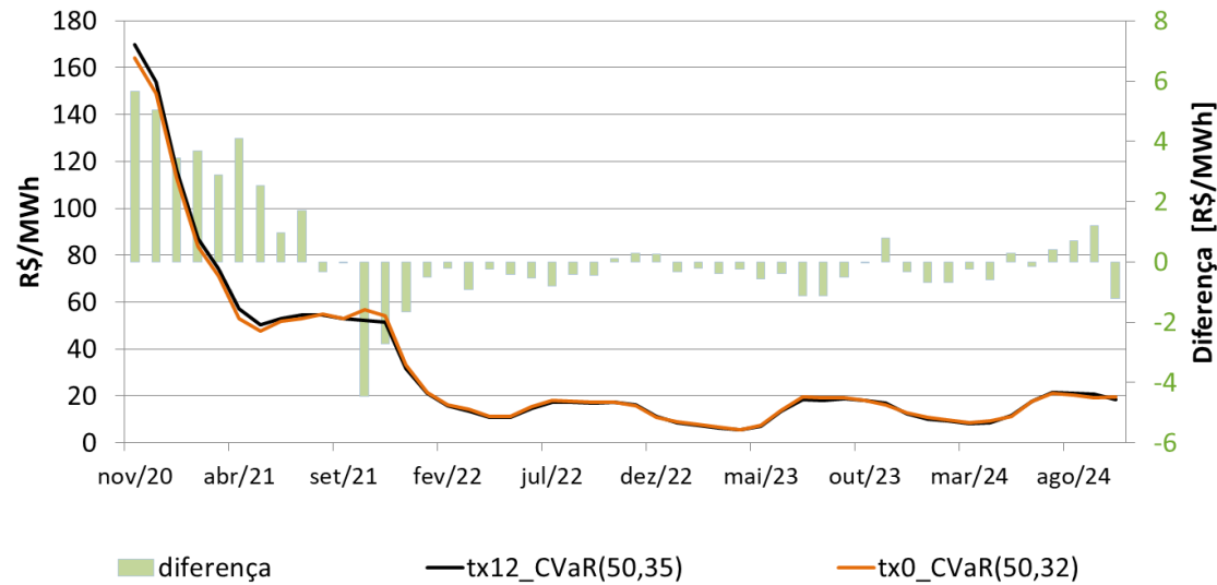
CMO - NORDESTE
