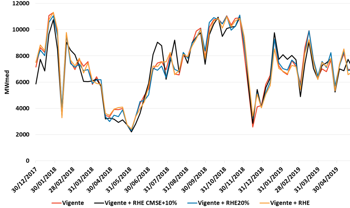
GH Sul
