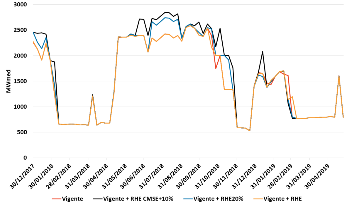
GT Norte
