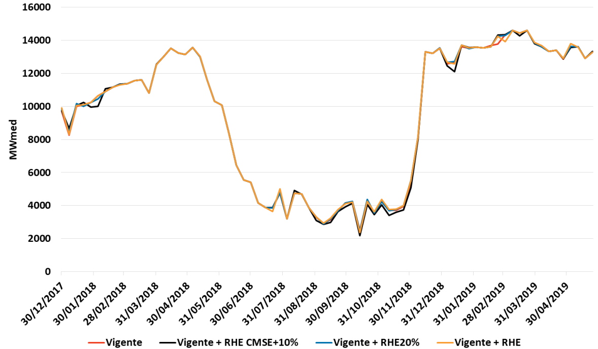
GH Norte
