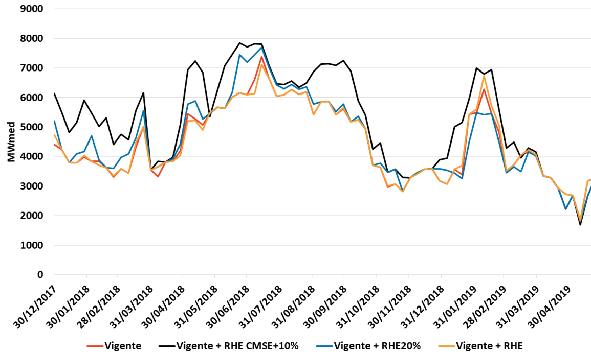
GT Sudeste
