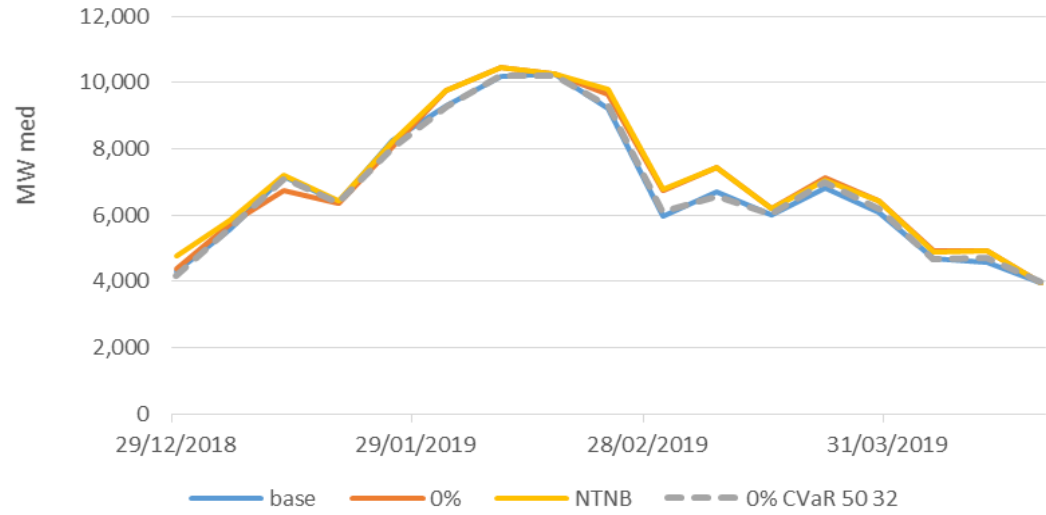
GT SIN
